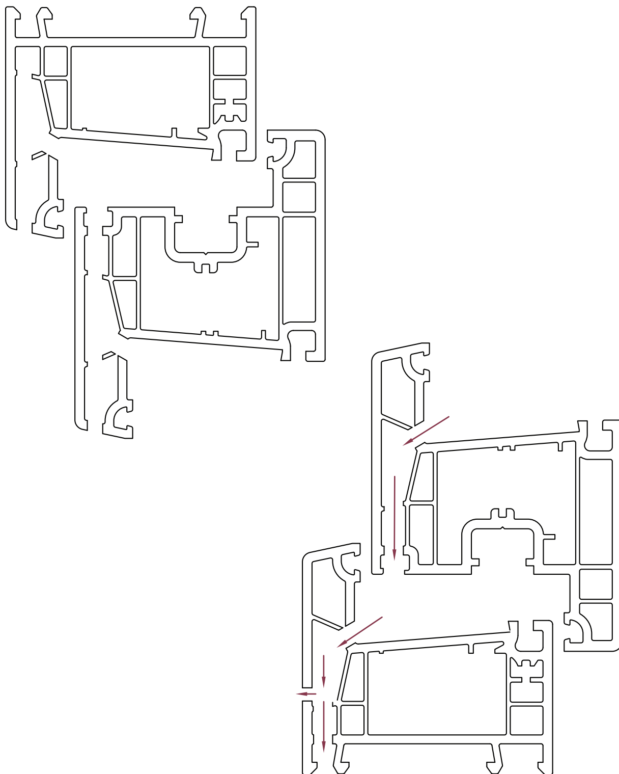
Водоотвод и вентиляция комбинации рама-створка (для белых профилей)
