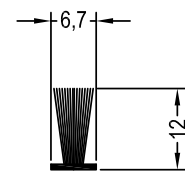
Щеточное уплотнение 6,7x12
