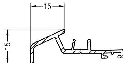
Слезник 15/70
